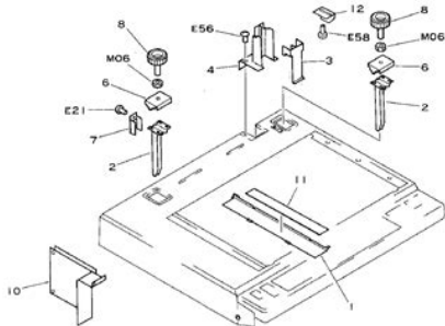
FIGURE 03 MOUNTING HARDWARE (NP-3525) 本体取付部品 (NP-3525)
